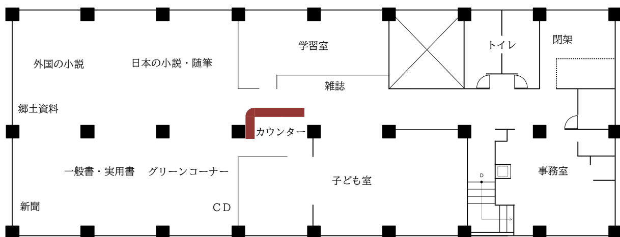
2階平面図
