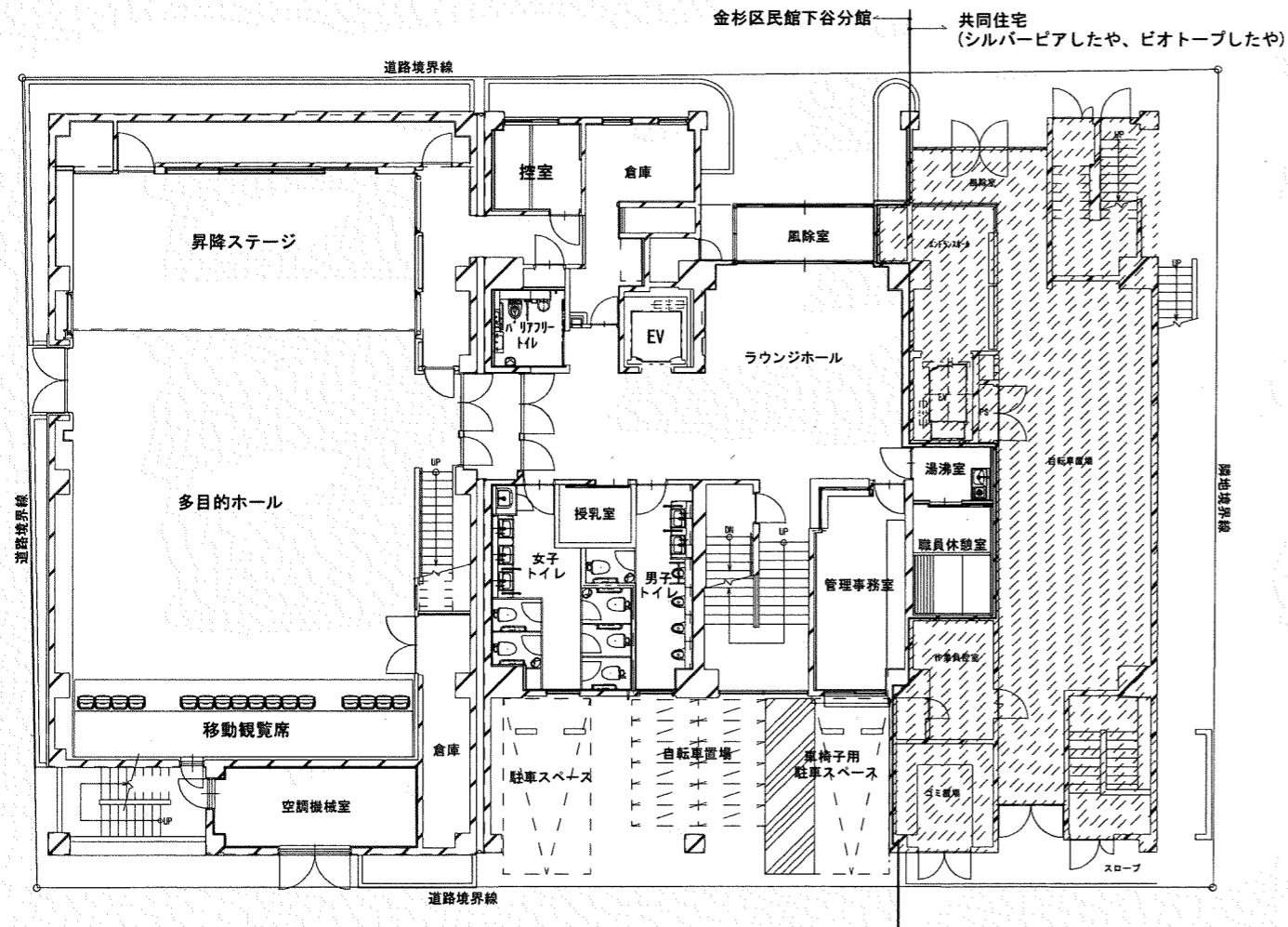
1階平面図
