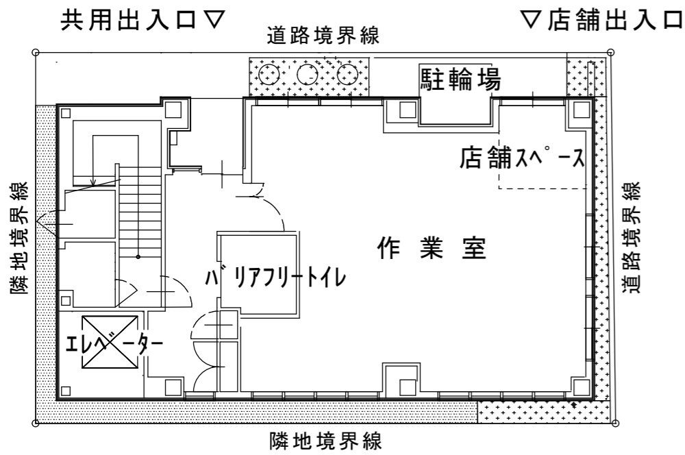
1階平面図 (福祉作業所)
