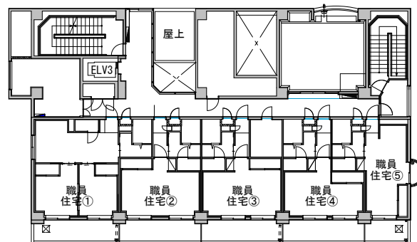
■ 7 階平面図
