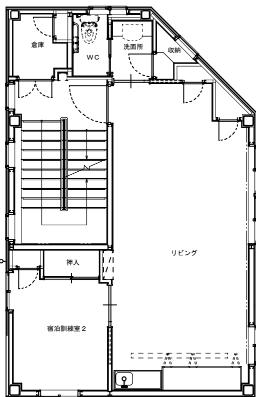
■ 2階平面図
