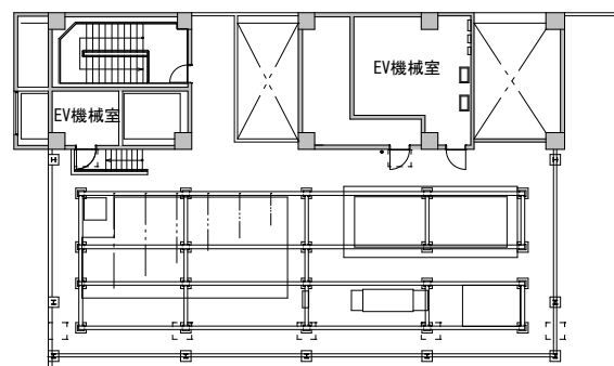
■ 塔屋階平面図
