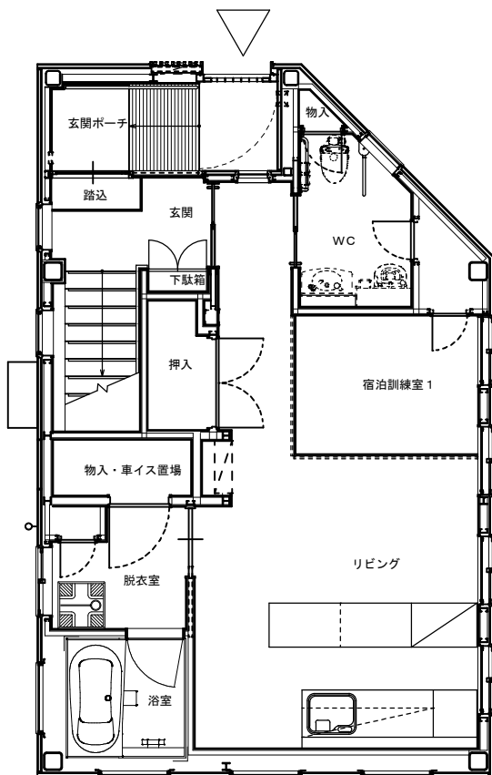
■ 1階平面図
