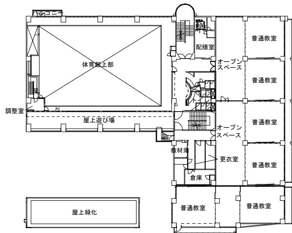
4階平面図
