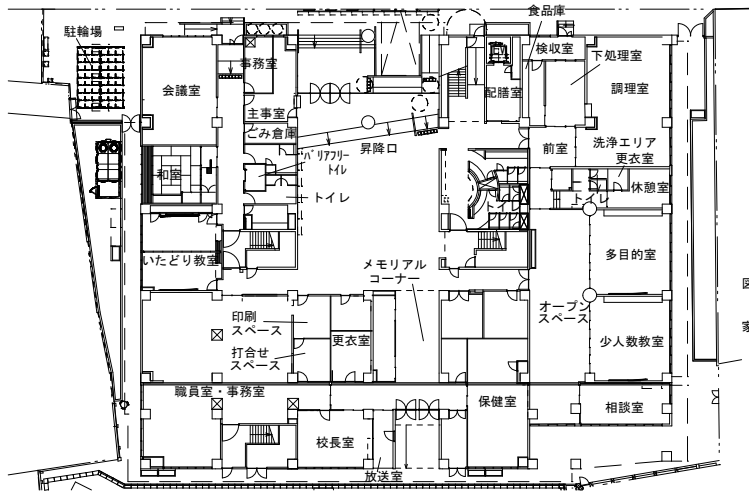
1階平面図
