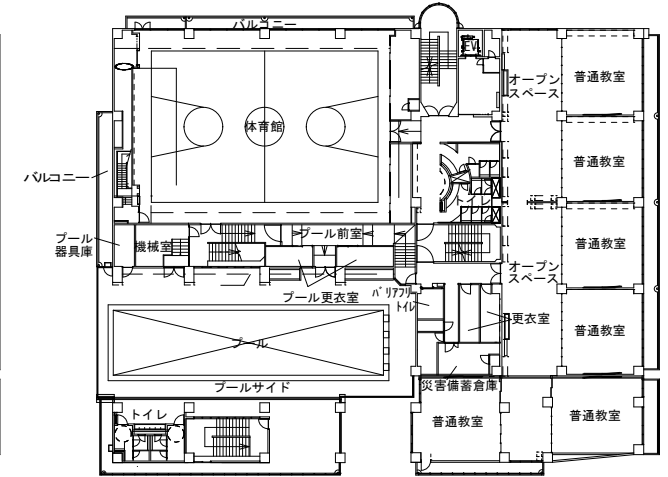
3階平面図
