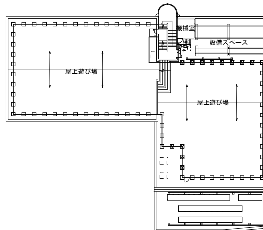
屋階平面図
