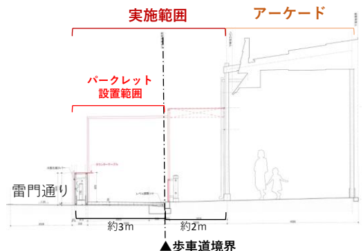
断面図
