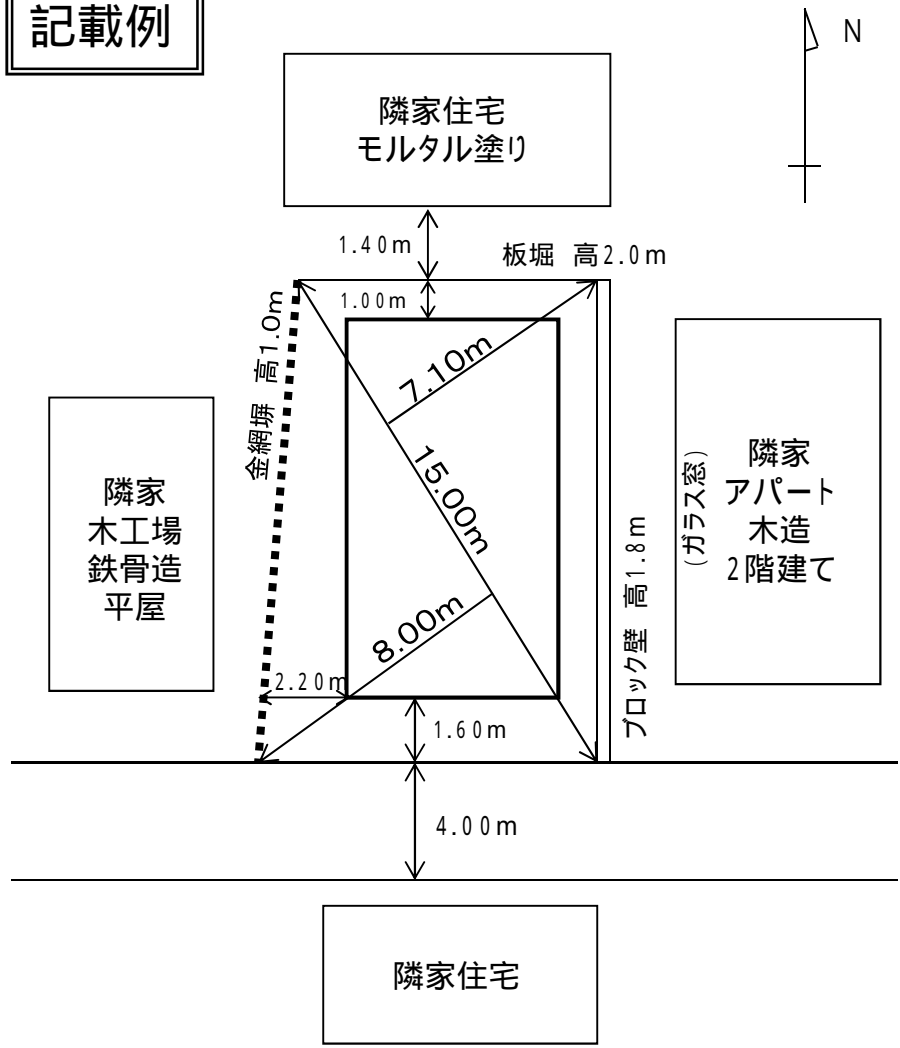
配置図 1/2000
