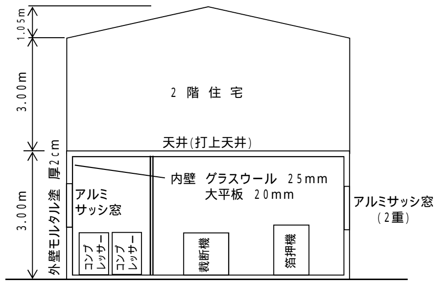
断面図 1/1000
