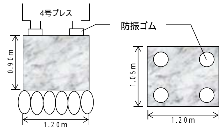
基礎断面図、平面図 1/300
