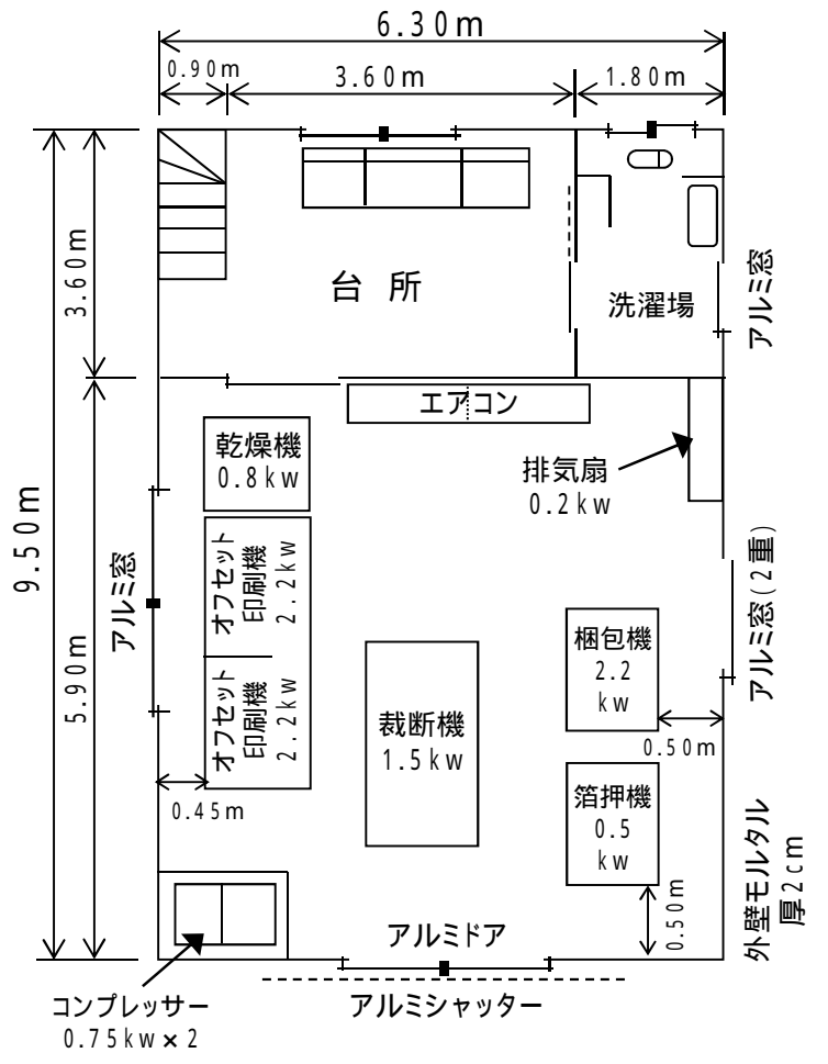
平面図 1/1000
