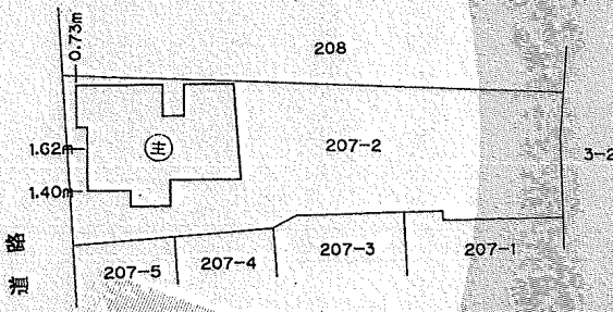
建物図面
