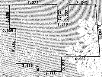
1階平面図 単位m
